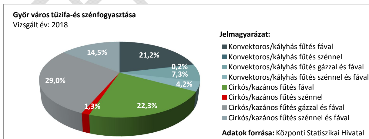
6. ábra: Lakossági tűzifa-és szénfogyasztásból származó szén-dioxid kibocsátás
