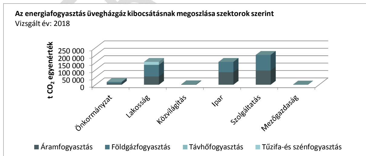
8. ábra: Győr energiafelhasználásának szektorok szerinti üvegházgáz kibocsátásának megoszlása
