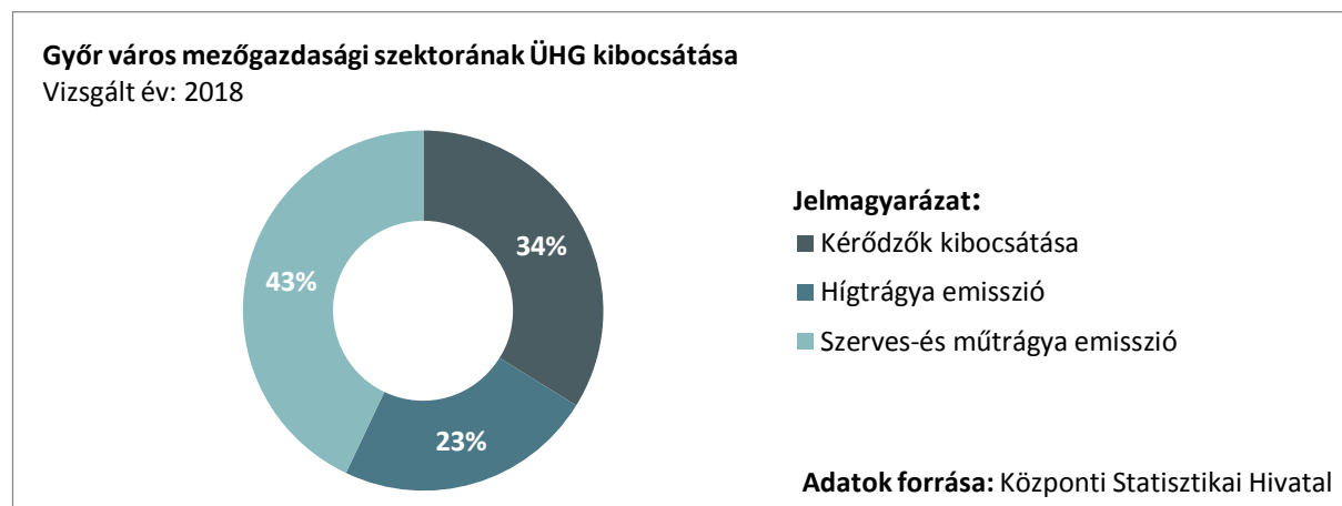
12. ábra: A győri mezőgazdaság CO 2 egyenértékre számított ÜHG kibocsátásának megoszlása
