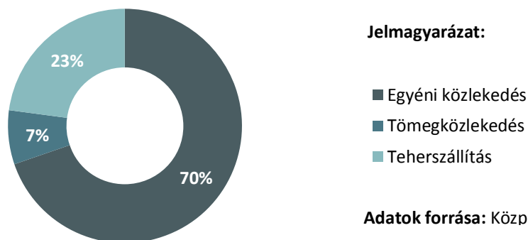
11. ábra: A CO 2 egyenértékben számított közlekedési ÜHG kibocsátás megoszlása
