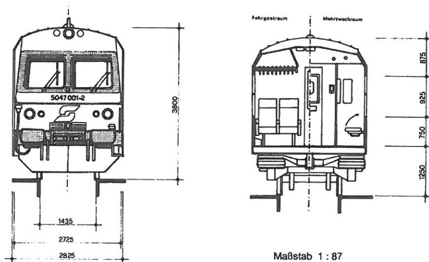
Homlokfal, keresztmetszet
