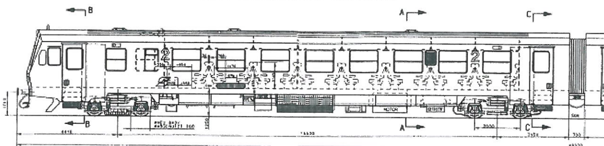
5047-es motorkocsi oldalnézete
