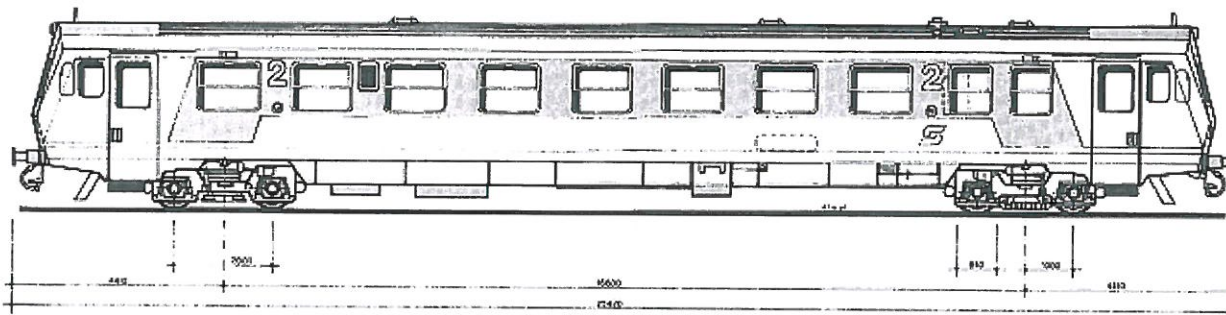
5047-es motorkocsi oldalnézete
