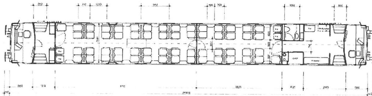
Alaprajz
