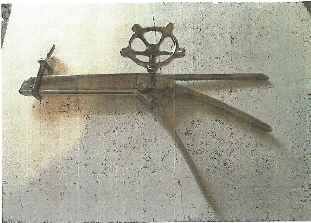
Petz-féle készülék operáció után, kapcsoló fogasléc kihúzva
