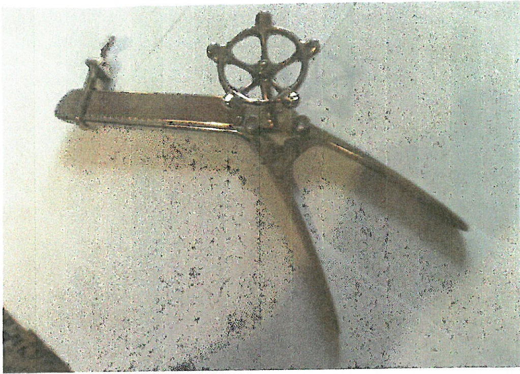
Petz-féle készülék operációra készen, kapcsoló fogasléc betolva
