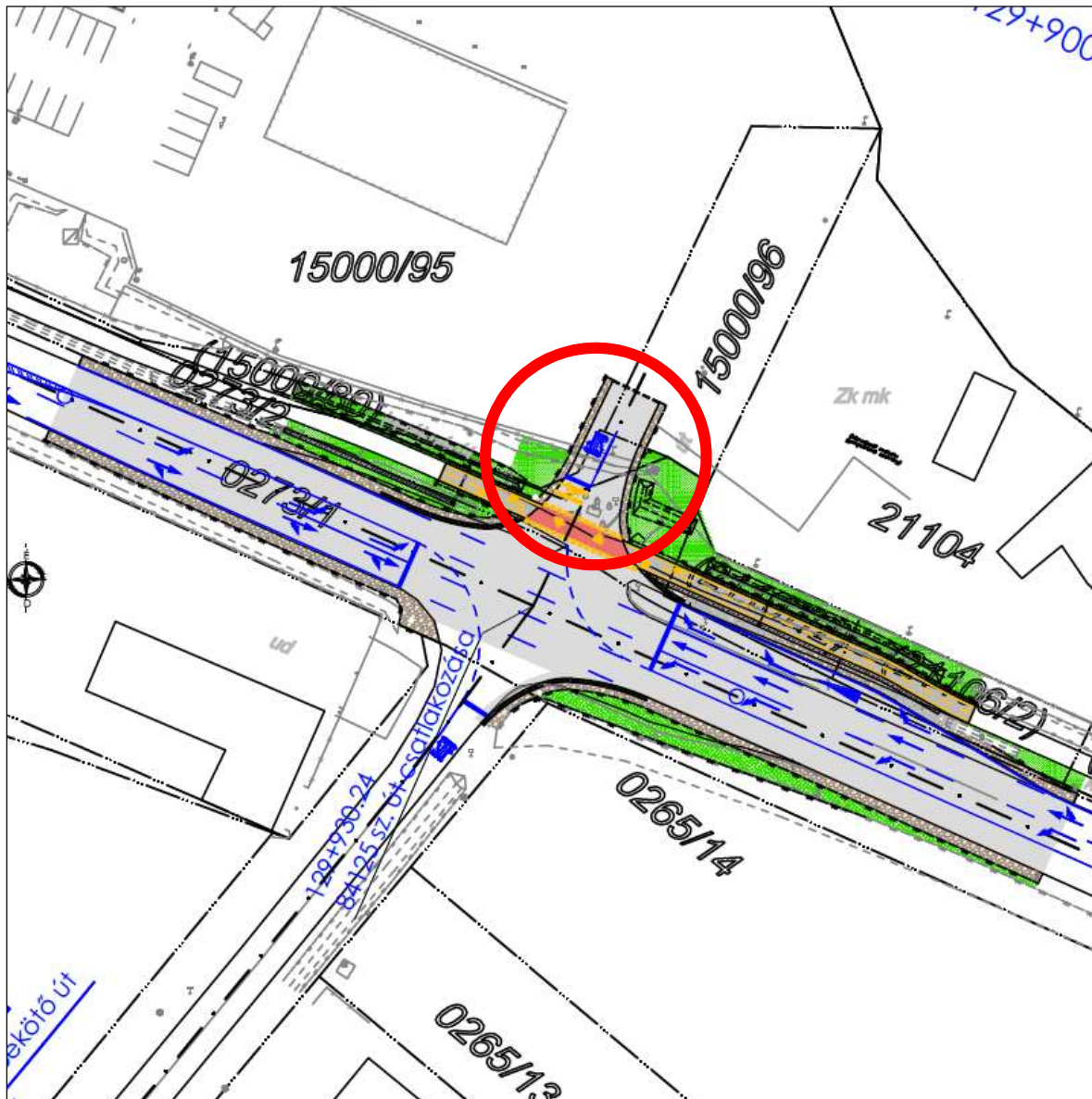
Kivágat az útengedélyezési kiviteli terv átnézeti helyszínrajzából (Pro Pervium Mérnöki Iroda Kft.)
